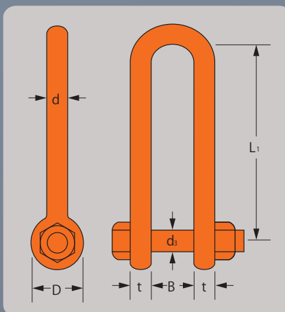
■寸法図
